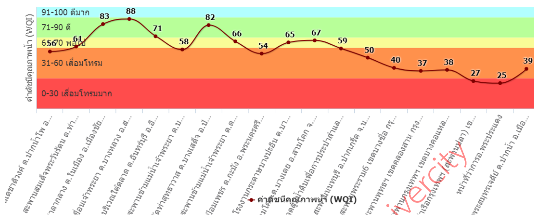
กราฟค่าดัชนีคุณภาพน้ำ (Water Quality Index) จุดตรวจวัดคุณภาพน้ำ แม่น้ำเจ้าพระยา
