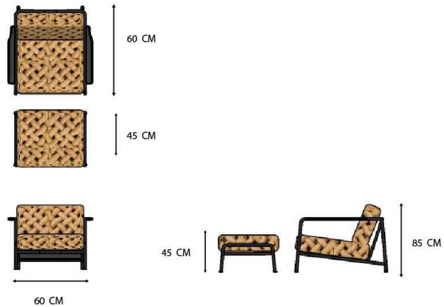
ภาพที่ 6 การเขียนแบบเพื่อการผลิต ผลิตภัณฑ์เก้าอี้จากเศษยางพาราแบบที่ 2
