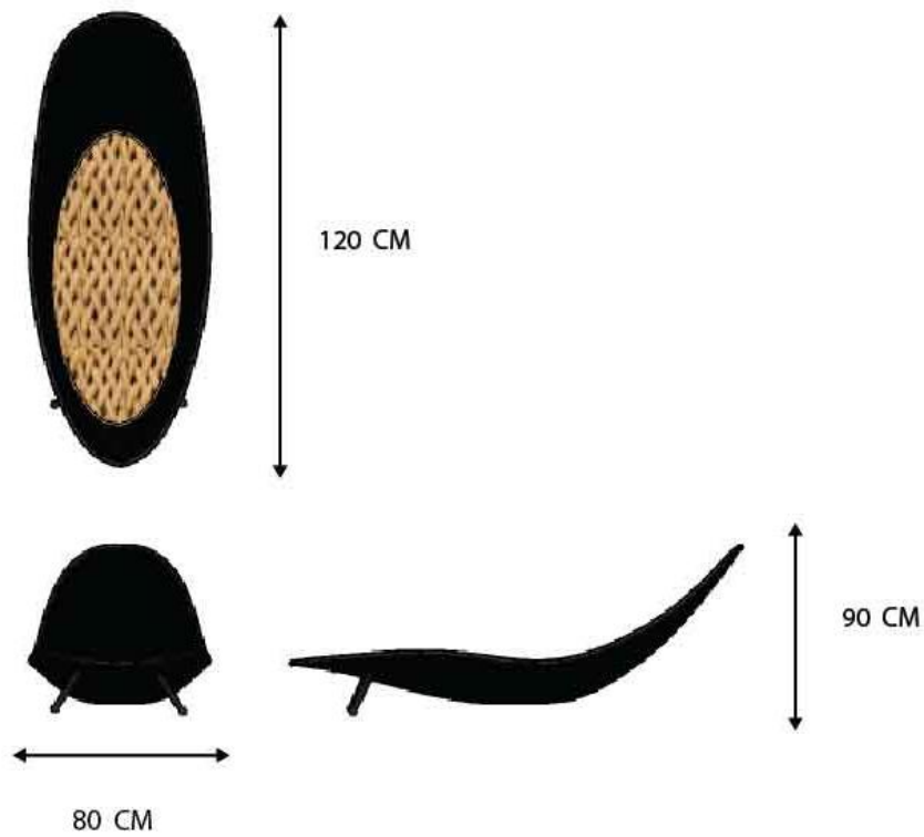
ภาพที่ 7 การเขียนแบบเพื่อการผลิต ผลิตภัณฑ์เก้าอี้จากเศษยางพาราแบบที่ 3
